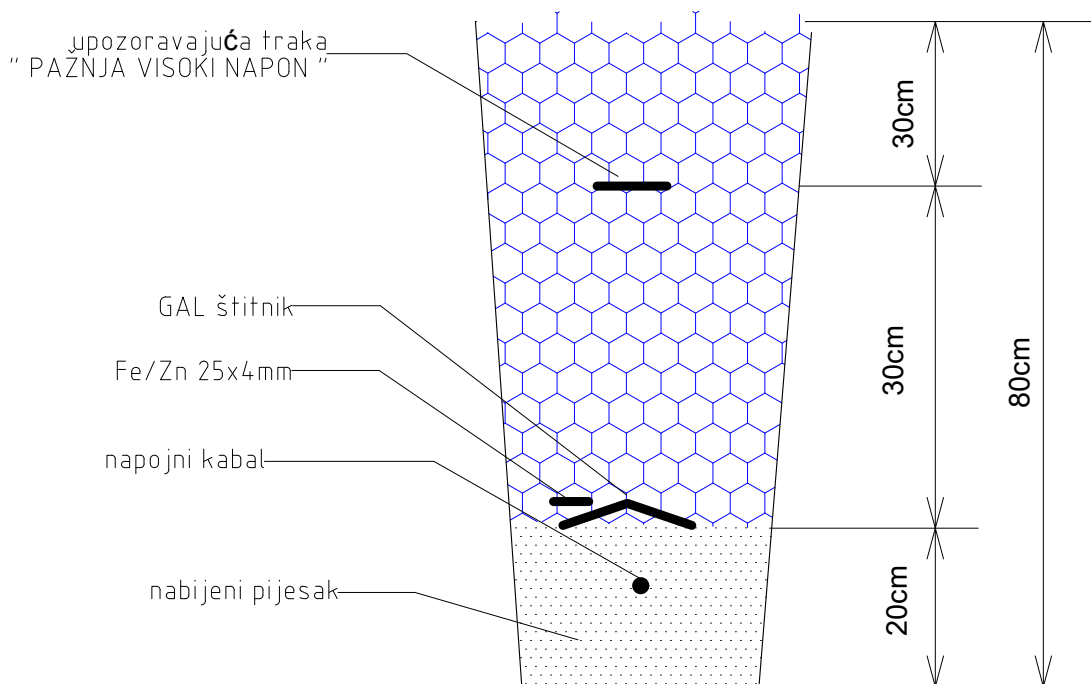
polaganje u slobodnom terenu
