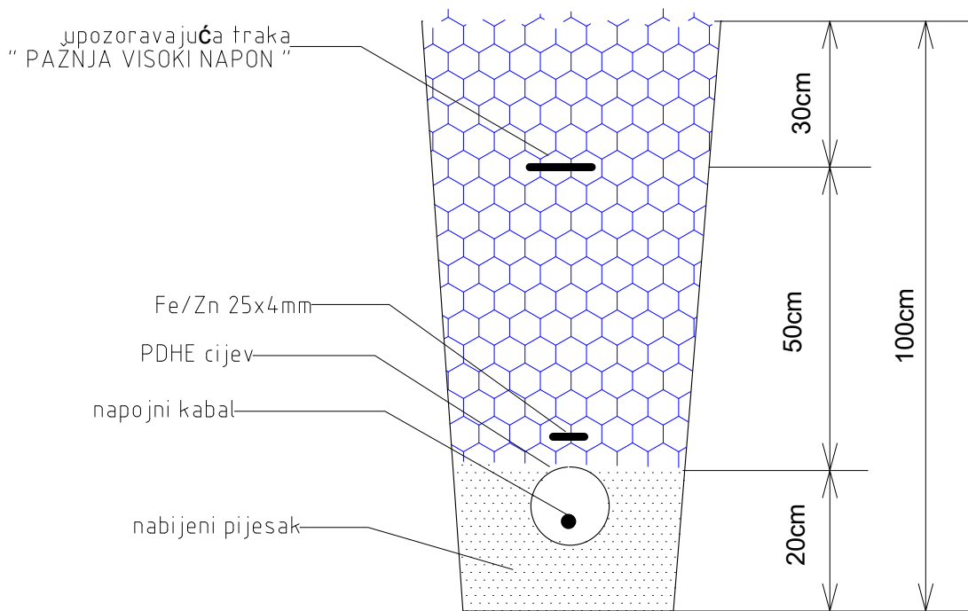
polaganje kablova ispod puta
