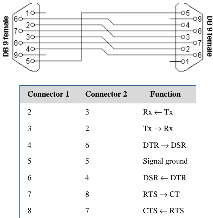
Slika 10. Serijska veza dva PC računara sa potpunim hardware handshake.
