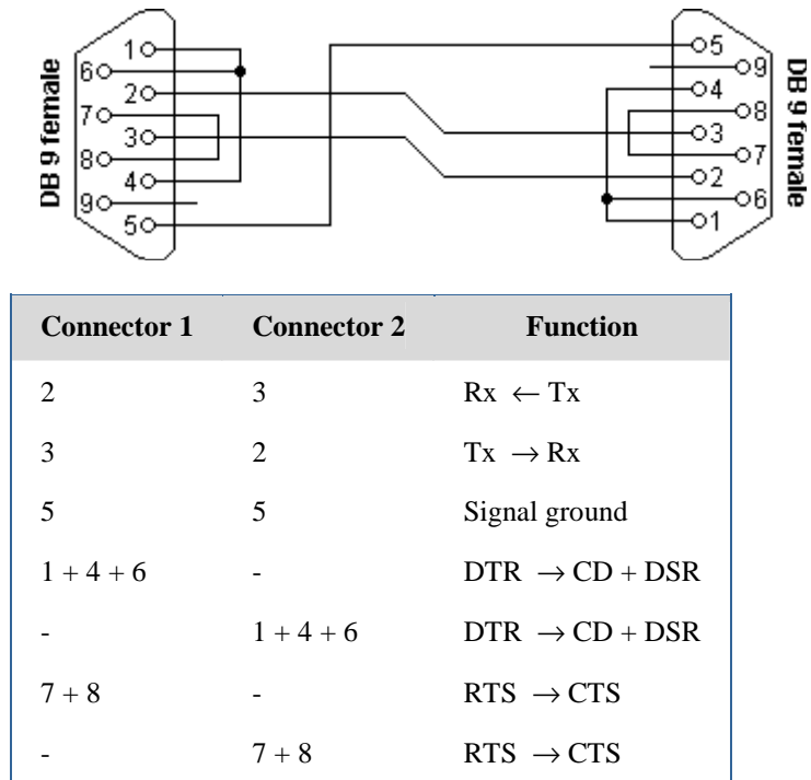
Slika 9. Serijska veza dva PC računara od kojih svaki ima svoj lokalni look back hardware handshake.
