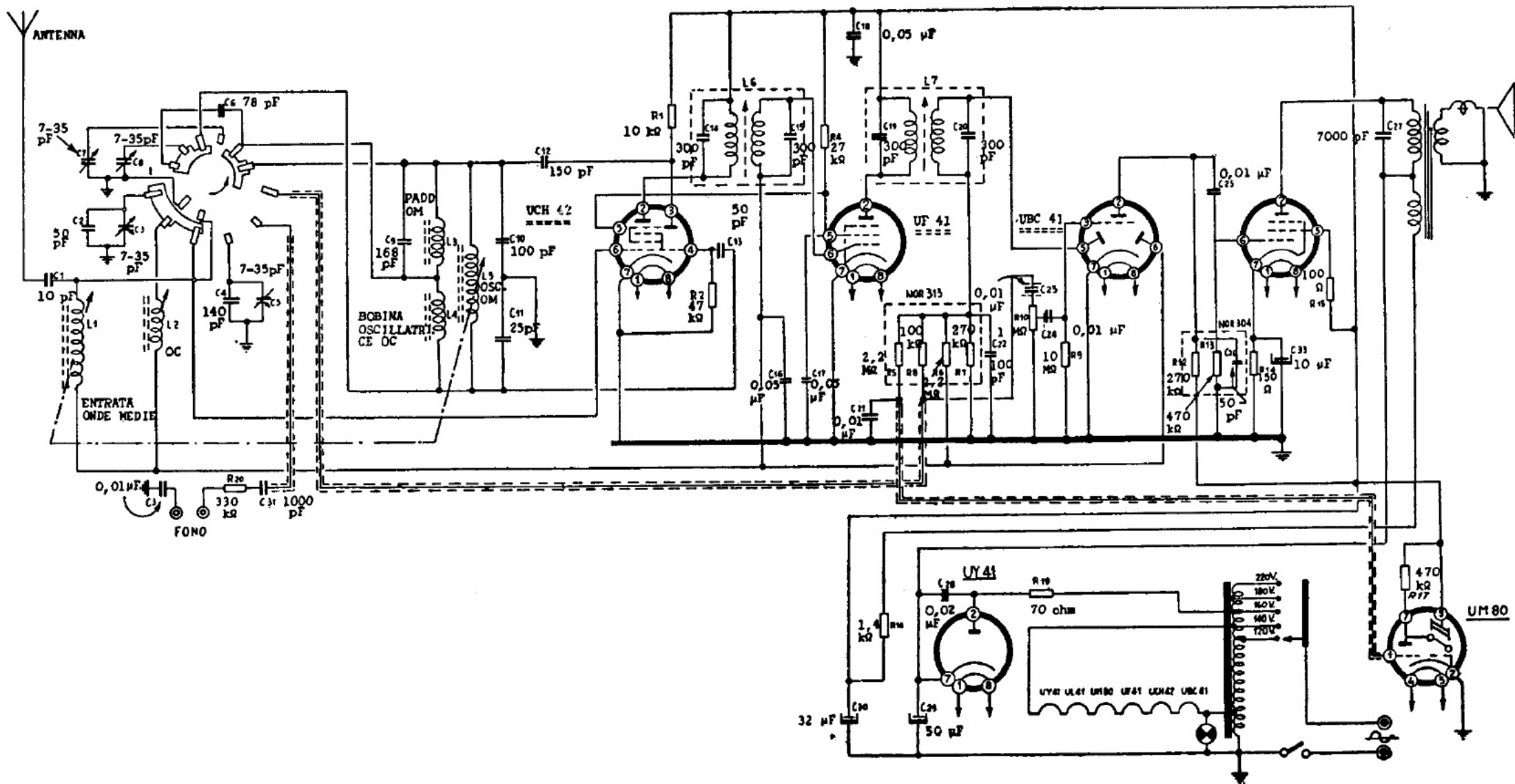
TELEFUNKEN RADIO TV - Mod. Telestar. Apparecchio con sintonia a permeabilità variabile. Gamma onde medic e due bande allargate a OC a 25 e a 50 metri. Media frequenza a 468 kc/s. Potenza d'uscita 1,5 watt.
