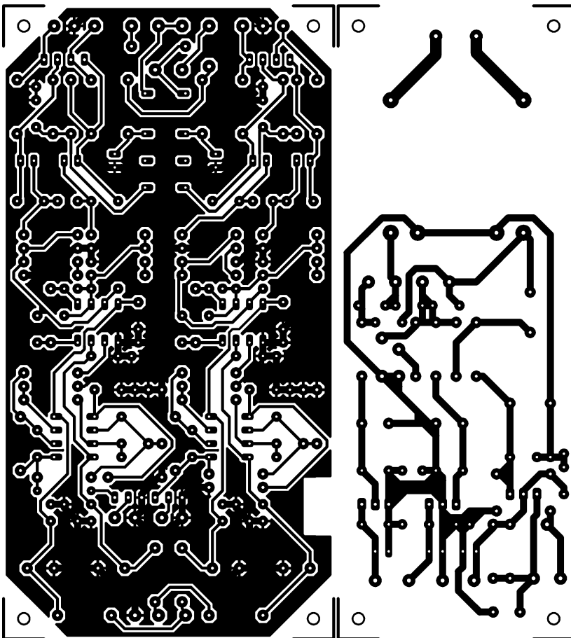
Mikrofonski stereo-pretpoja~ava~
