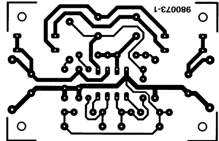
DC-DC pretvara~
