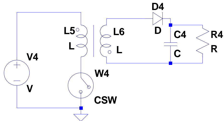
4) jos malo "prevrtanja" i imamo klasican flyback
