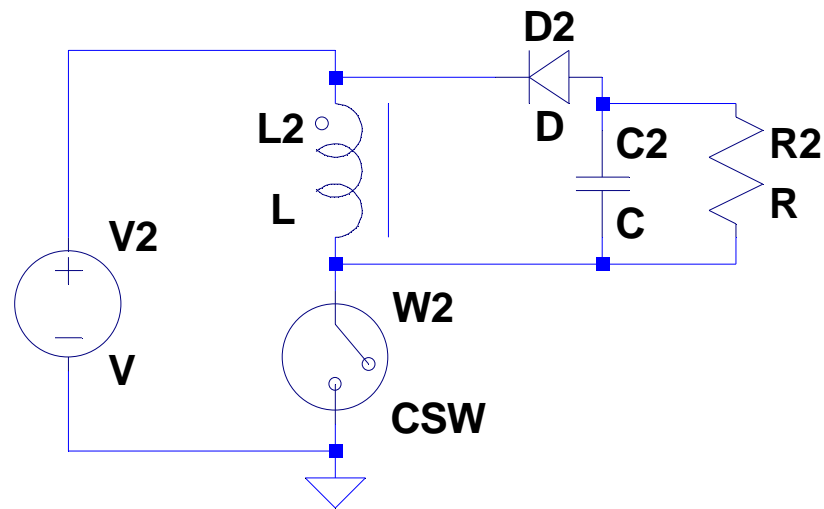
2) isto, samo malo prevrnuto
