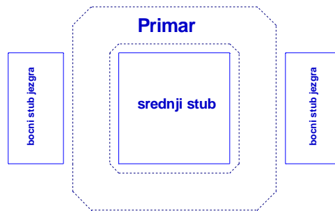
Presek, pogled odozdo (sa strane primara)
