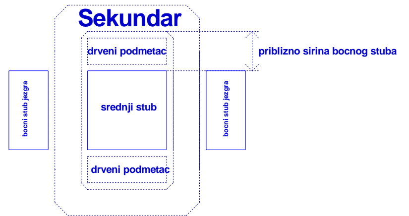
Presek, pogled odozdo (sa strane sekundara)
