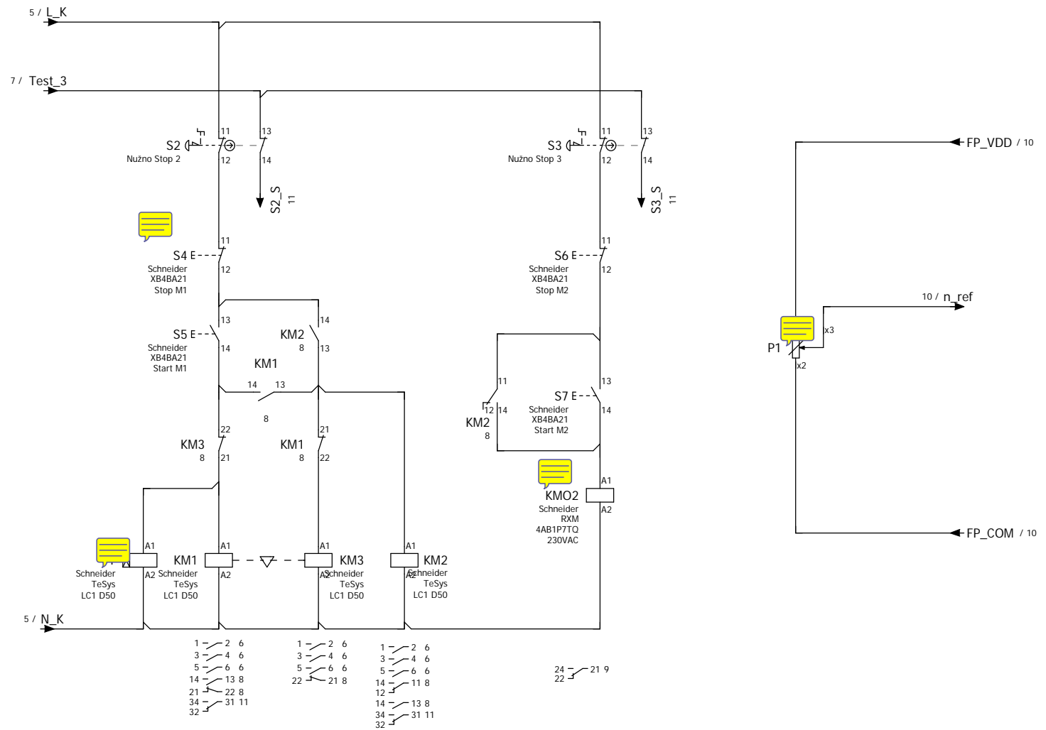
Kontrola motora 1
