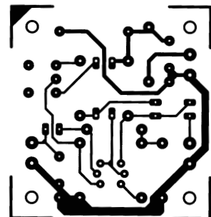
Mikrofonski pretpoja~ava~
