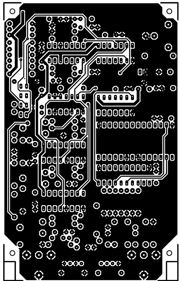
Jednostavan eliminator Copybit-a
