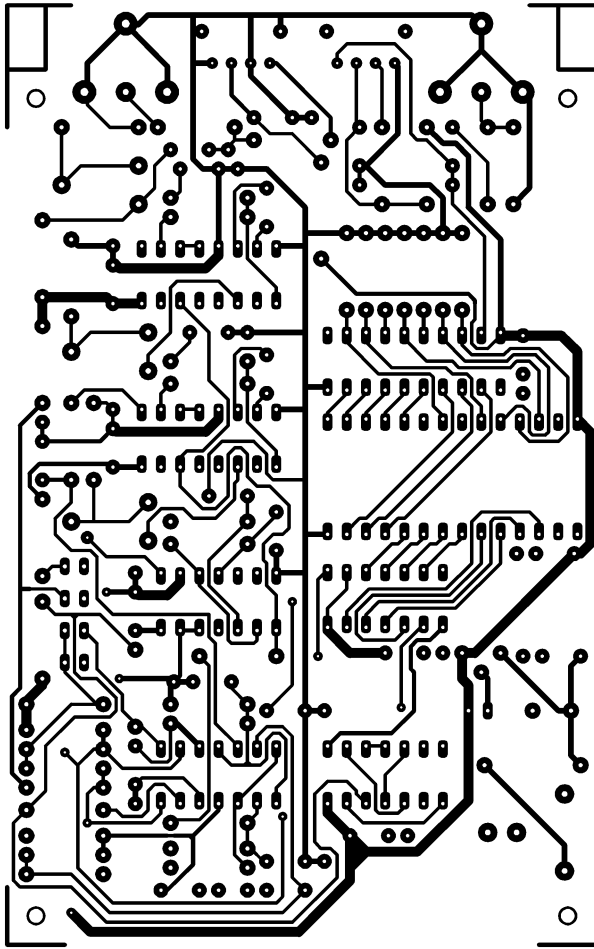
Jednostavan eliminator Copybit-a
