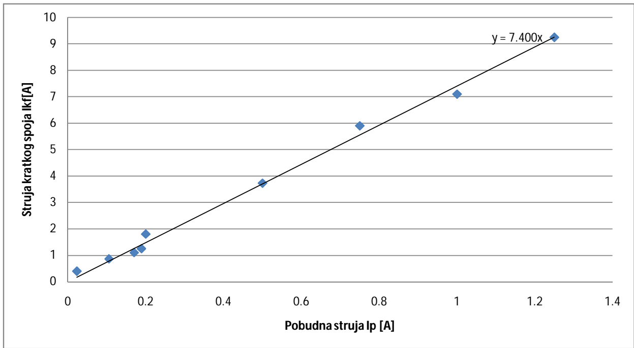
Karakteristika kratkog spoja
