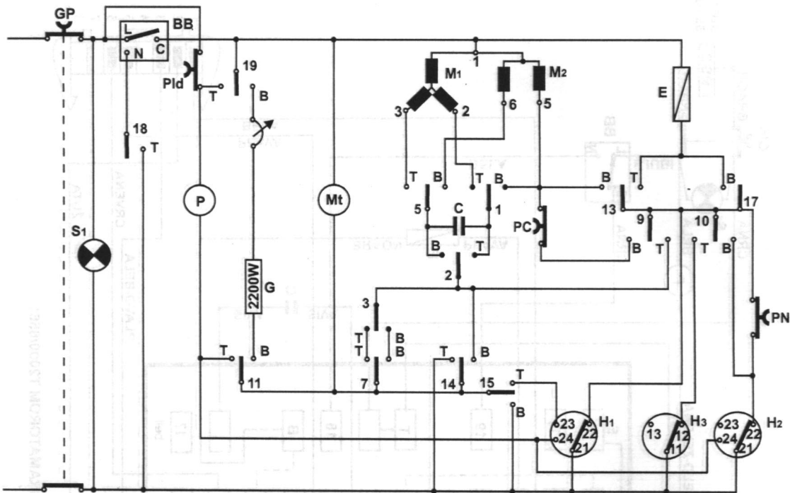
ELEKTRIČNA ŠEMA VEŠ MAŠINA WA 543 I WA 583 SA PROGRAMATOROM T2000 / 6561
