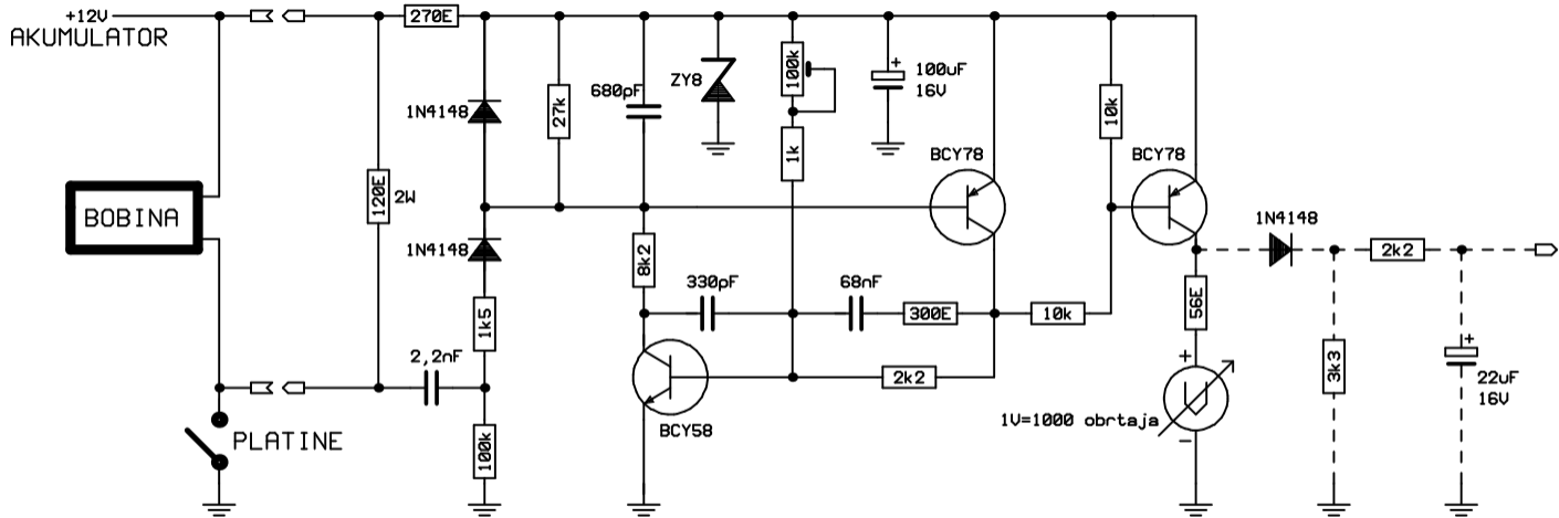
ANALOGNI OBRTOMER
