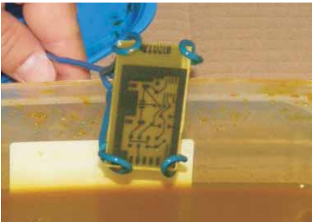
13. Pločica je izgrizena
