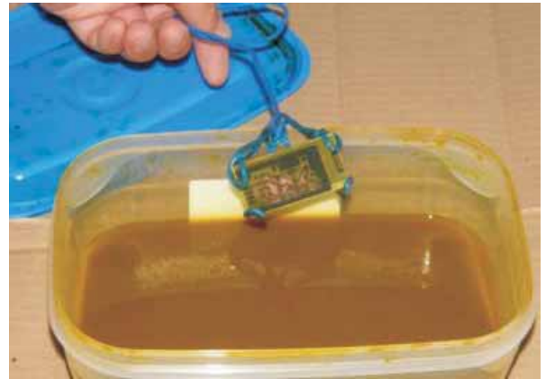
12. Uranjanje u medij za nagrizanje. Povremeno malo protresti, da se postupak ubrza.
