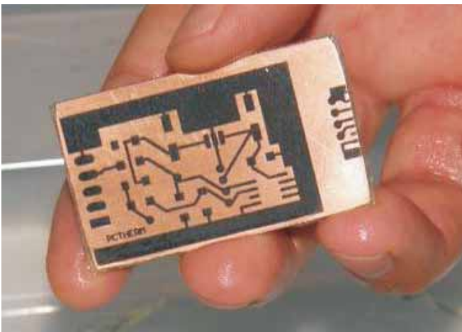
9. Isprana pločica spremna za nagrizanje.
