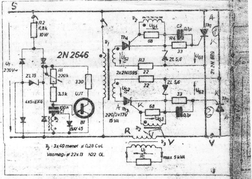
8.4. ábra. Antiparallel tirisztorpár vezérlése „széles” impulzusgenerátorral
