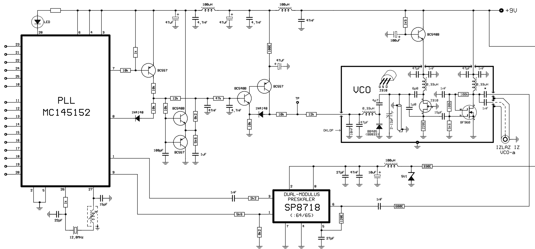
Univerzalni PLL-sintisajzer za VHF i UHF sa razmakom kanala od 25KHz Dizajn: Dr. Borivoje Jagodić YZ10XB
