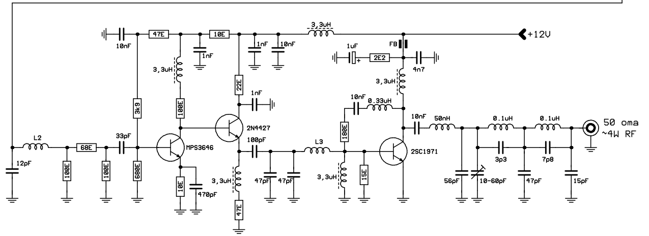
88-108MHz FM STEREO ENCODER ( 100KHz raster ) Dizajn: Dr. Borivoje Jagodic YZ10XB
