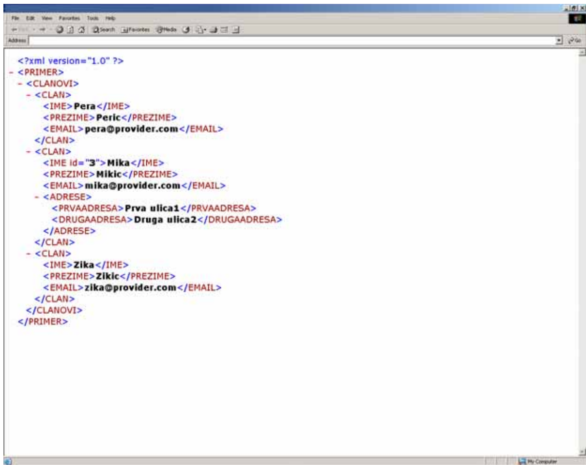
Slika 2 izgled parsiranog fajla u pretraživaču
